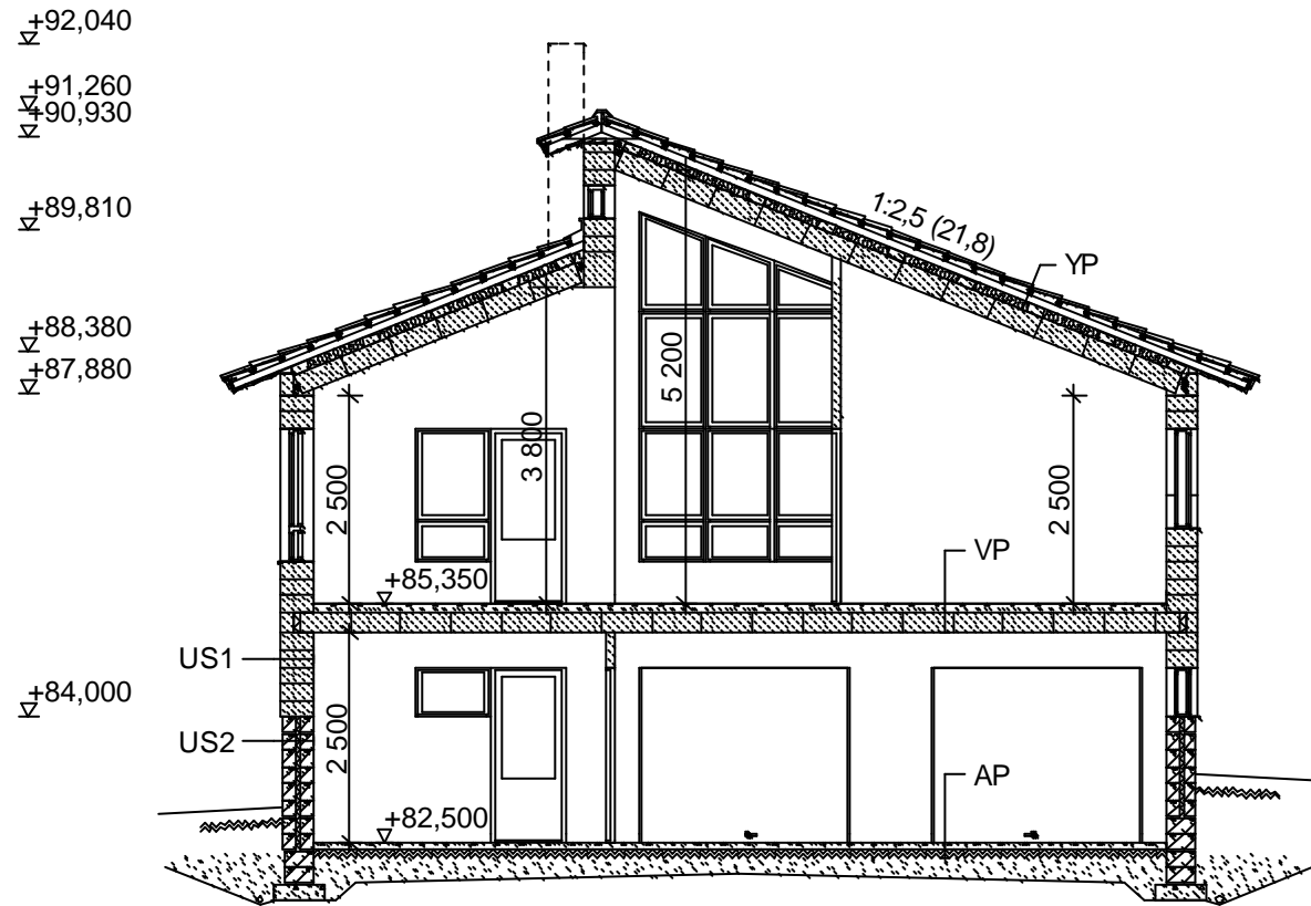
LEIKKAUS A-A
