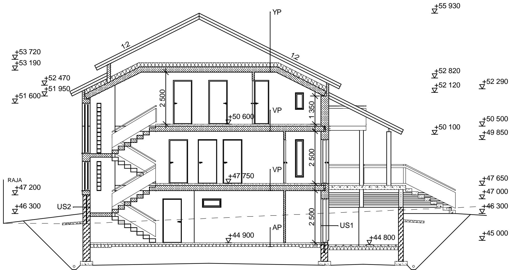
LEIKKAUS B-B
