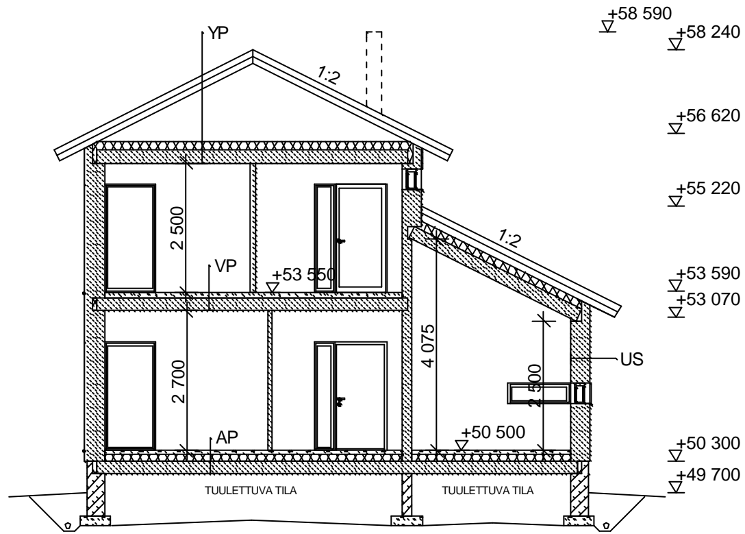
LEIKKAUS A-A
