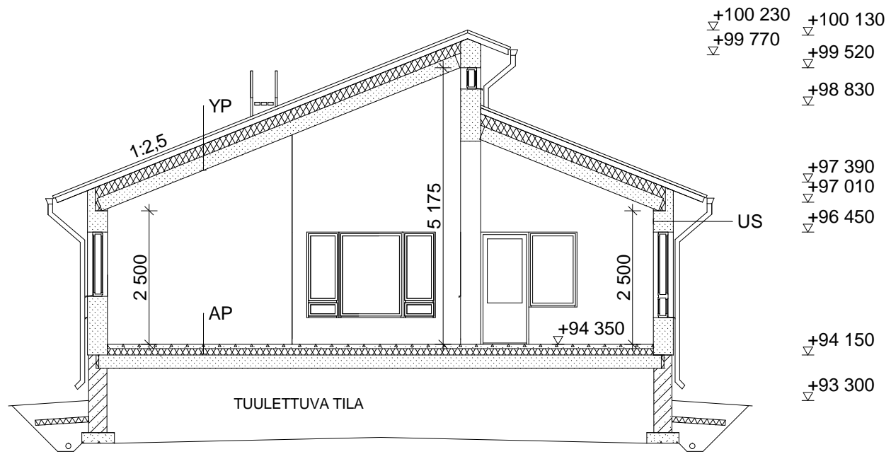
LEIKKAUS A-A
