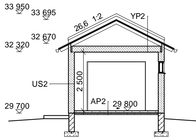
LEIKKAUS B-B
