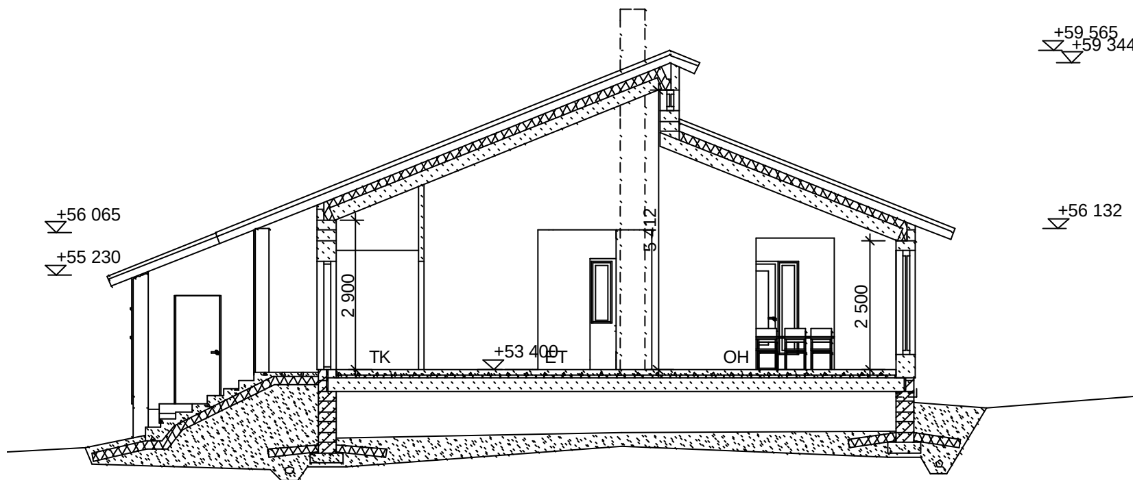
LEIKKAUS A-A
