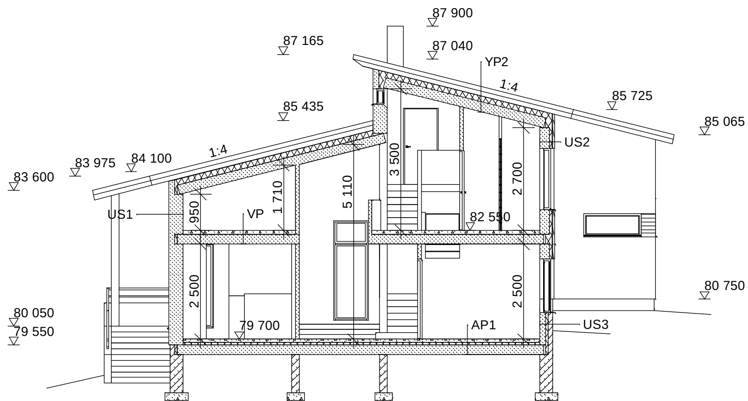
LEIKKAUS B-B
