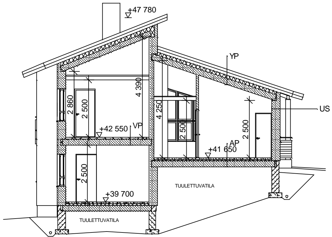
LEIKKAUS A-A
